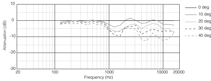
垂直离轴频率响应 (向下):
