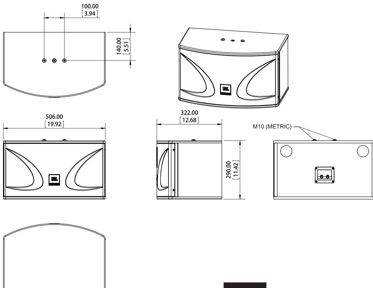
外形尺寸 单位: mm (inch/ 英寸)
