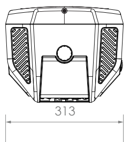
Onderaanzicht
