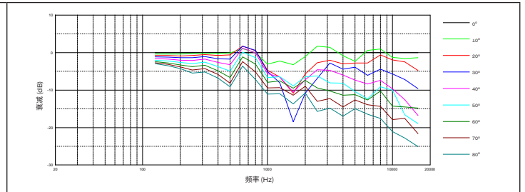
垂直离轴频率响应:
