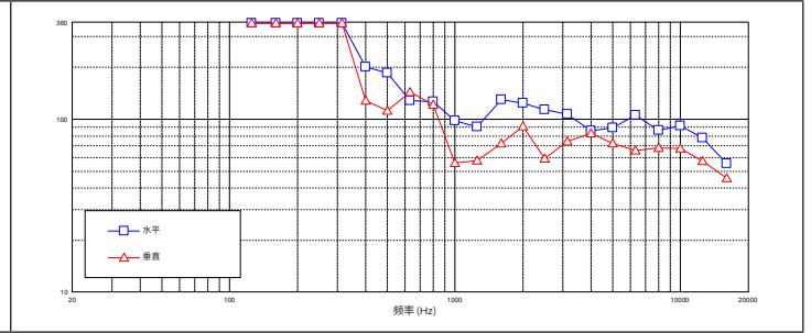
垂直离轴频率响应:
