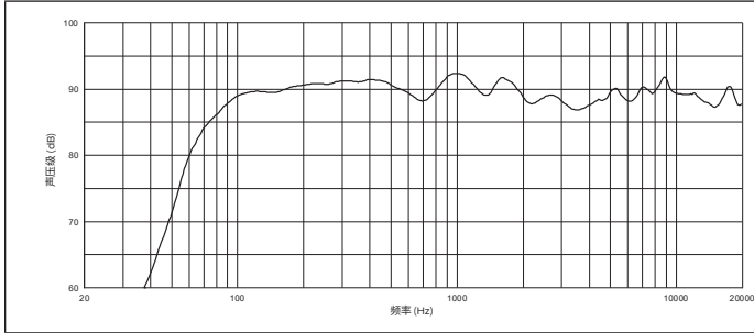
水平离轴频率响应:
