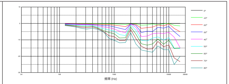
垂直离轴频率响应:
